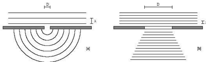
Figura 2.3: Effetto della diffrazione nei casi \lambda > D in [a] e \lambda < D in [b]
