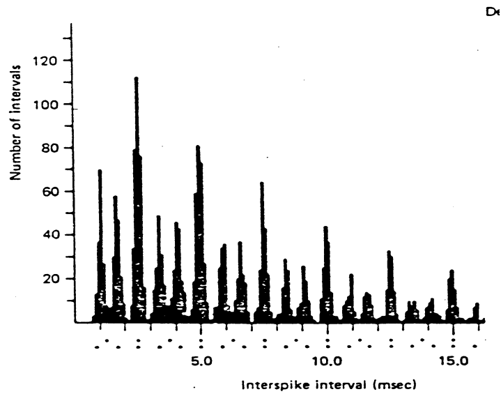
Figura 2.23: Istogramma del numero di occorrenze di dato tempo di intercorrenza fra spike successivi nel nervo uditivo a fronte di un'eccitazione composta da due suoni puri
