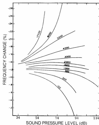
Figura 2.11: Diagramma di Stevens e Wolkmann (1937). Variazione del pitch di una sinusoide in funzione dell'intensità. Una sinusoide di 150 Hz passando da 45 a 90 dB scende in pitch del 12%, circa di due semitoni. Una curva discendente implica che la frequenza del suono deve essere aumentata per avere la stessa sensazione di pitch.
