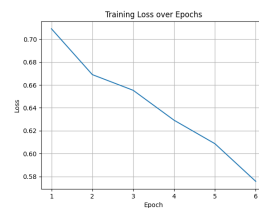
(d) BERT-large
