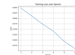
(d) BERT-large
